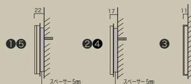
鏡面仕上げのステンレスをシャープに曲げたエッジ
